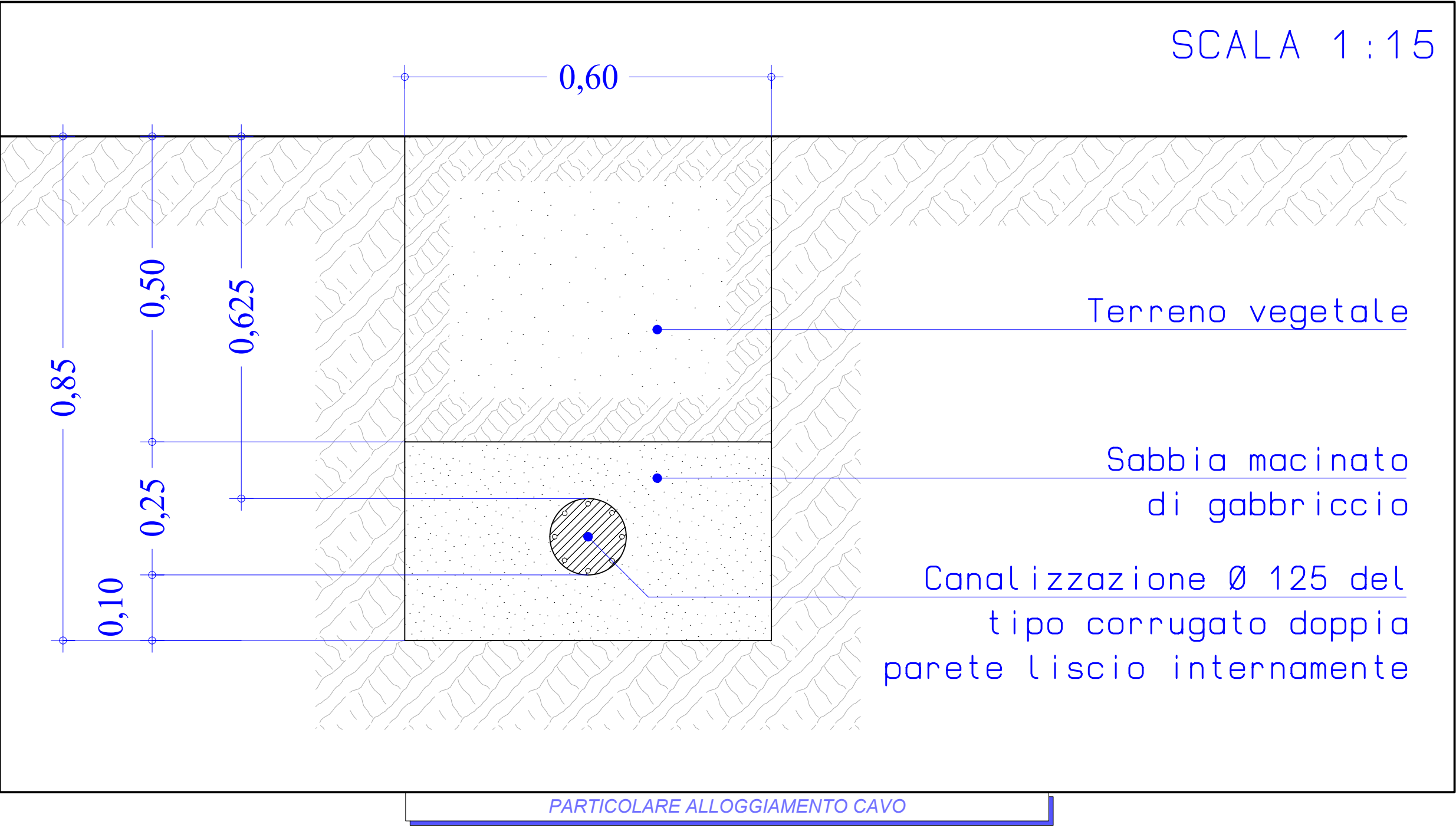
PARTICOLARE ALLOGGIAMENTO CAVO
