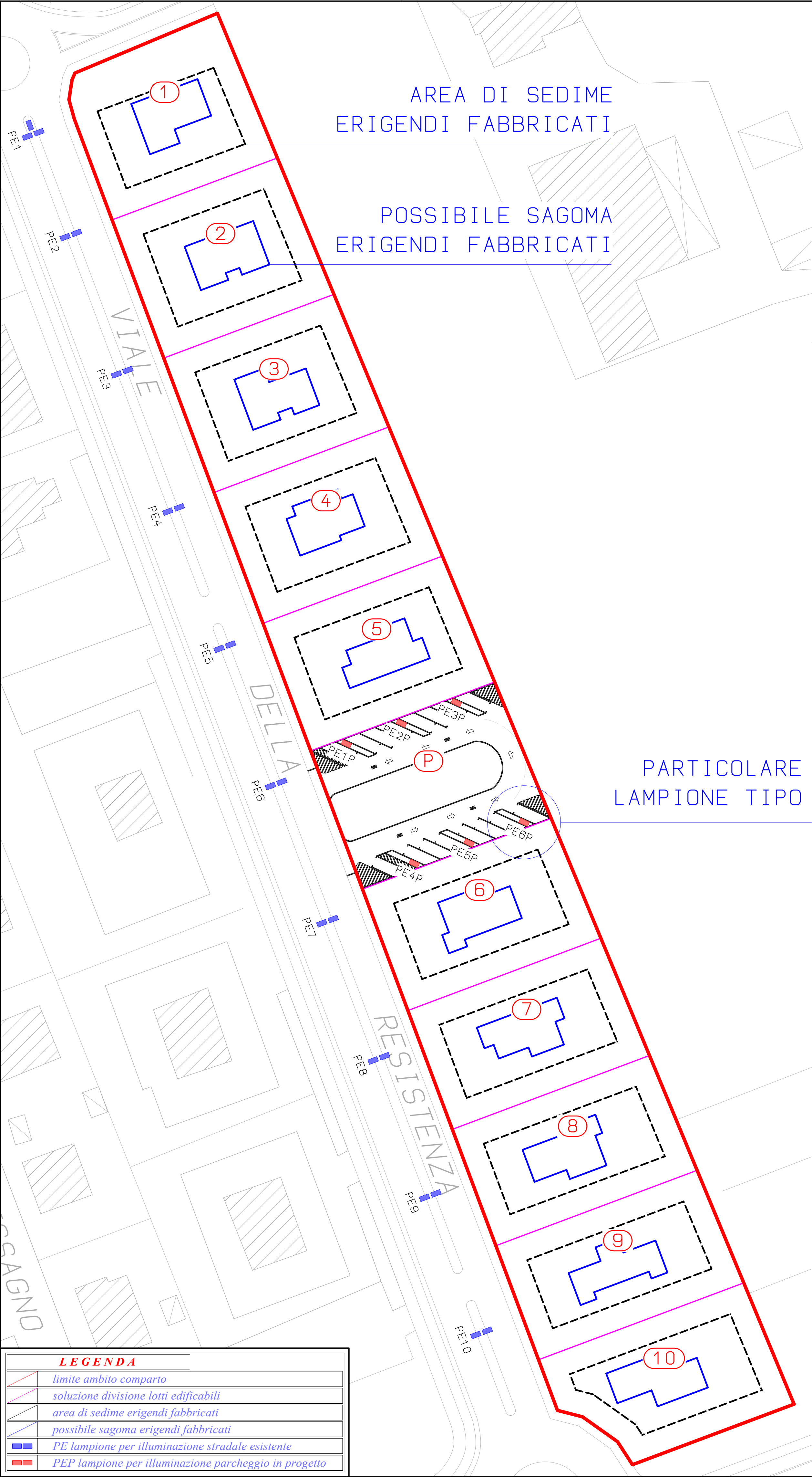
PLANIMETRIA GENERALE LOTTI EDIFICABILI
