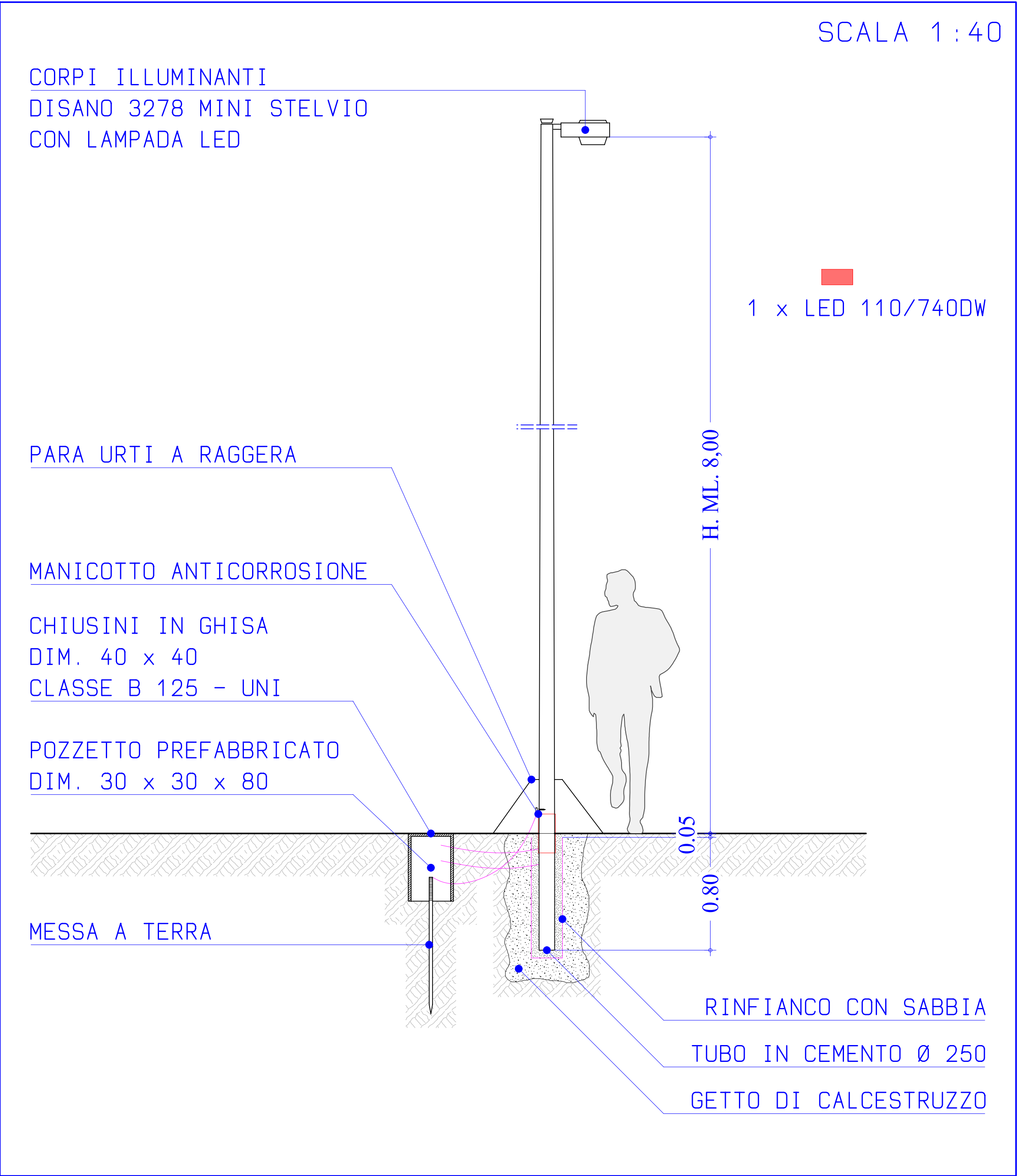
PARTICOLARE LAMPIONE DI PROGETTO
